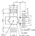
PCB板腳位焊盤 (5:1)
