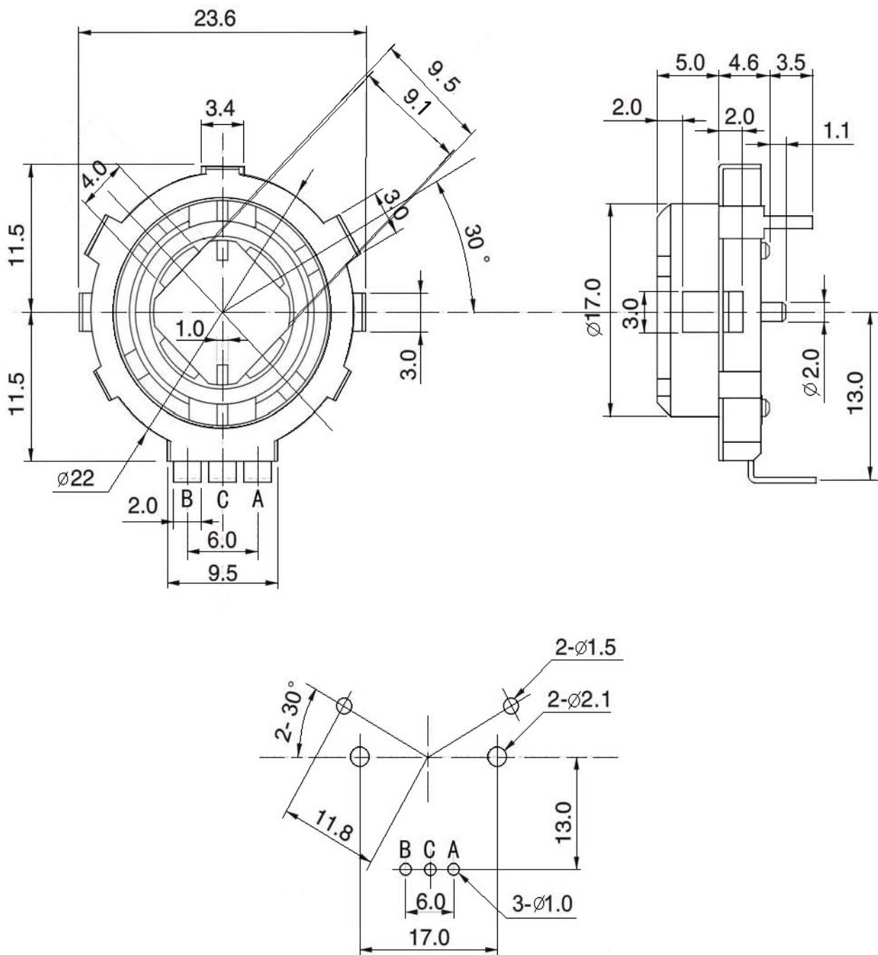
線路板安裝詳細尺寸 P.C.B mounting detail
