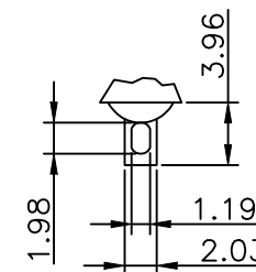
SOLDER LUG
