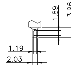
SOLDER LUG
