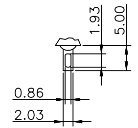
SOLDER LUG
