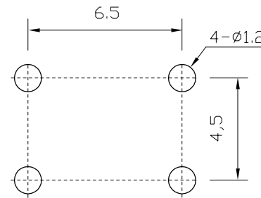
P.C.B HOLE
