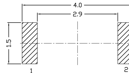
PCB. 焊接图
